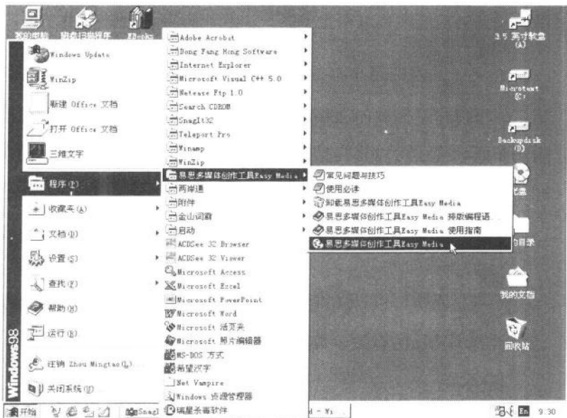
图 1-6 “开始”菜单
