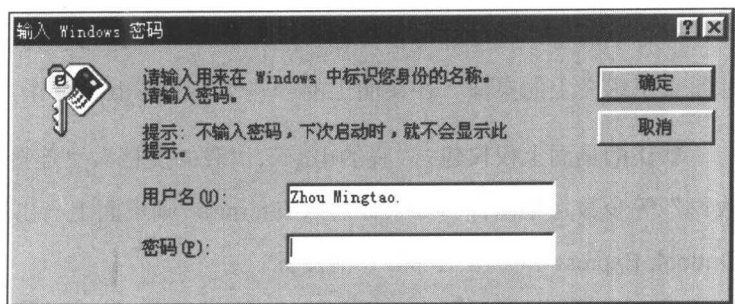
图 1-3 登录对话框
