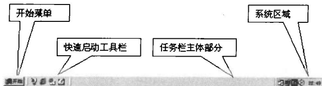
图 1-5 任务栏
