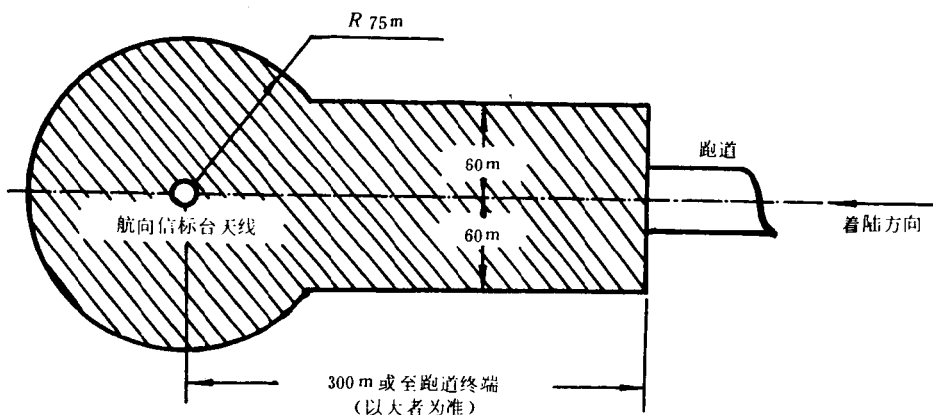
图 2 航向信标台保护区
