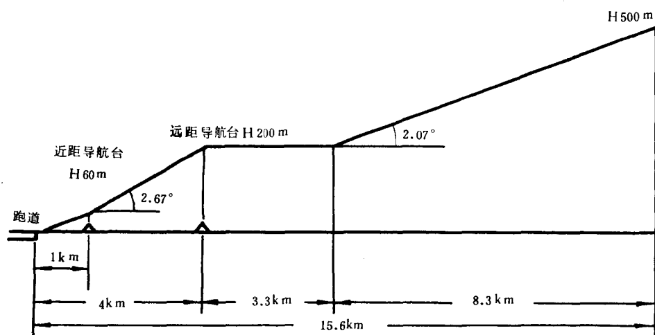
飞机下滑线
