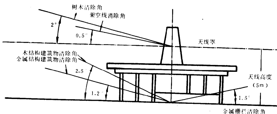
图7 全向信标台场地要求
