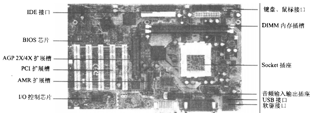
图 1-3 Socket 主板
