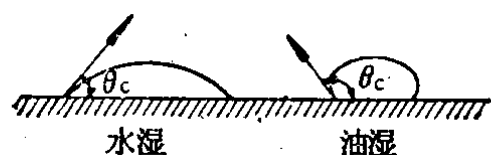
图 2-1 油-水-固体系统的润湿性 [8]
