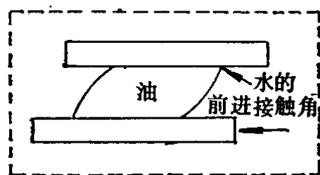
图 2-2 接触角的度量
