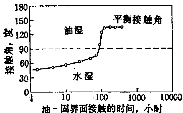
图 2-3 趋于平衡的接触角
