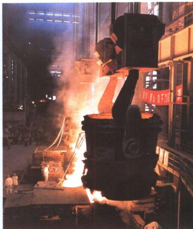
1992 年中国钢铁产量突破 8000 万吨。图为中国最大的大型轧机机架在首都钢铁公司浇铸成功。 ——宋连峰 摄
