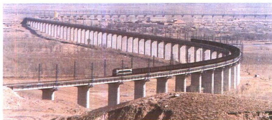
1992 年大同一秦皇岛铁路全面通车。图为列车通过永定河大桥 ——贲兰武 摄
