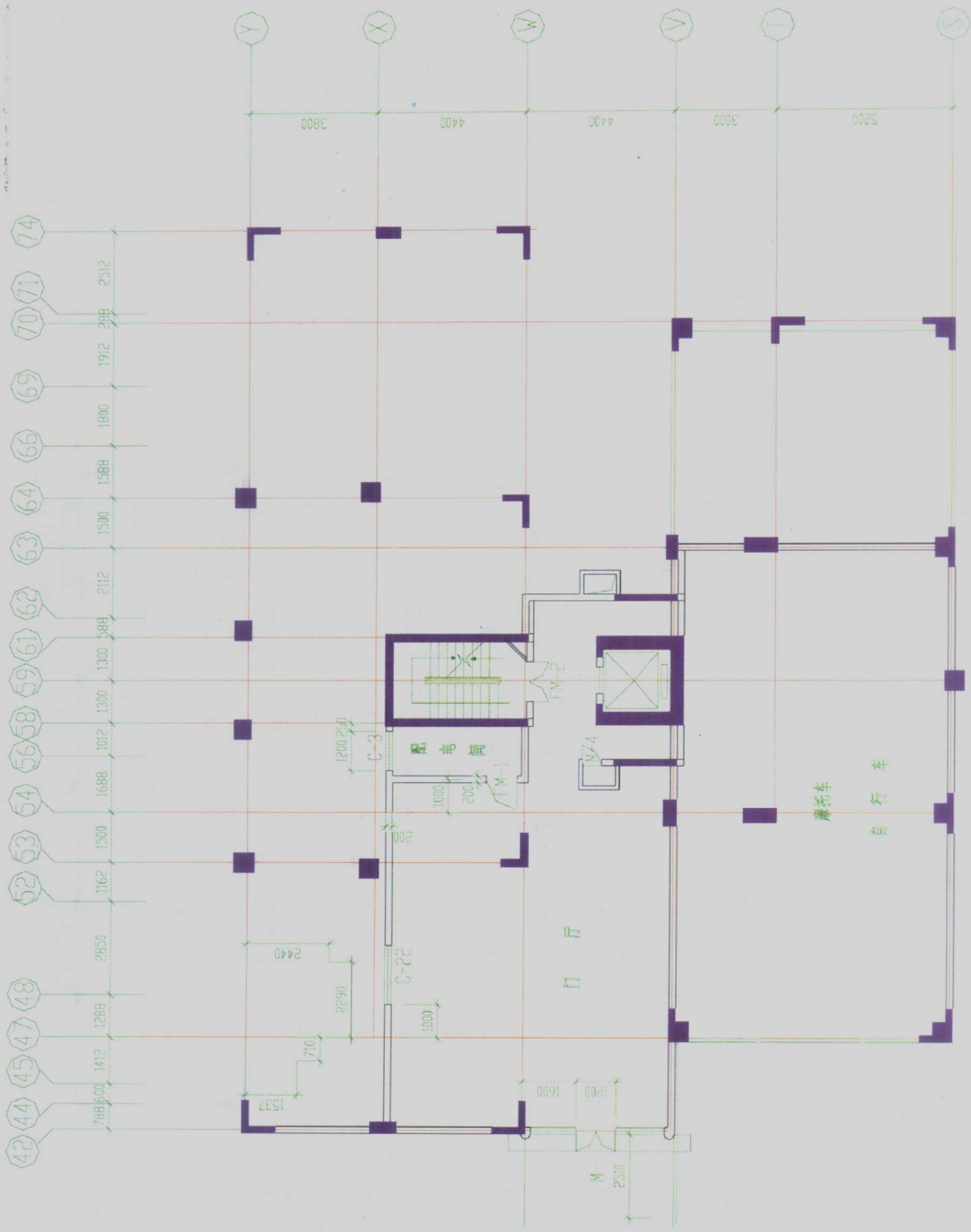
底层平面图
