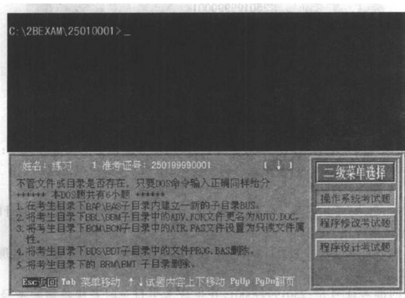
图 1.1.7 考试画面
