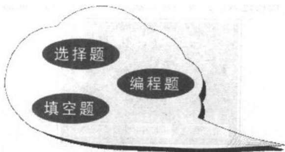
图 1.2.5 “题型”显示
