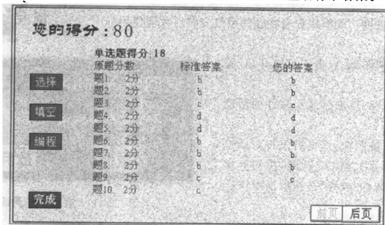
图 1.2.7 “判卷”界面
