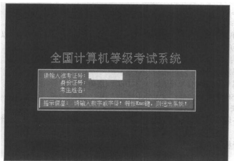
图 1.1.2 登录画面
