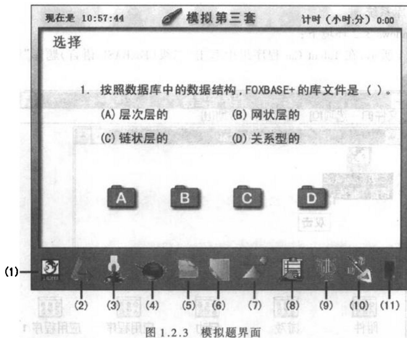
图 1.2.3 模拟题界面
