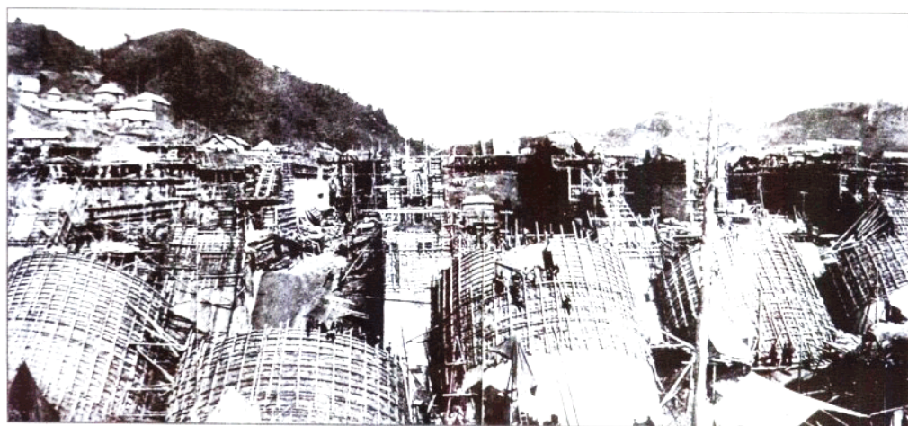
1953 年施工中的佛子岭水库连拱坝
