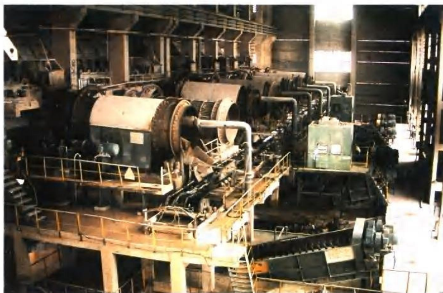
镇江船山石灰石矿洗矿车间的圆筒和槽式洗矿机
