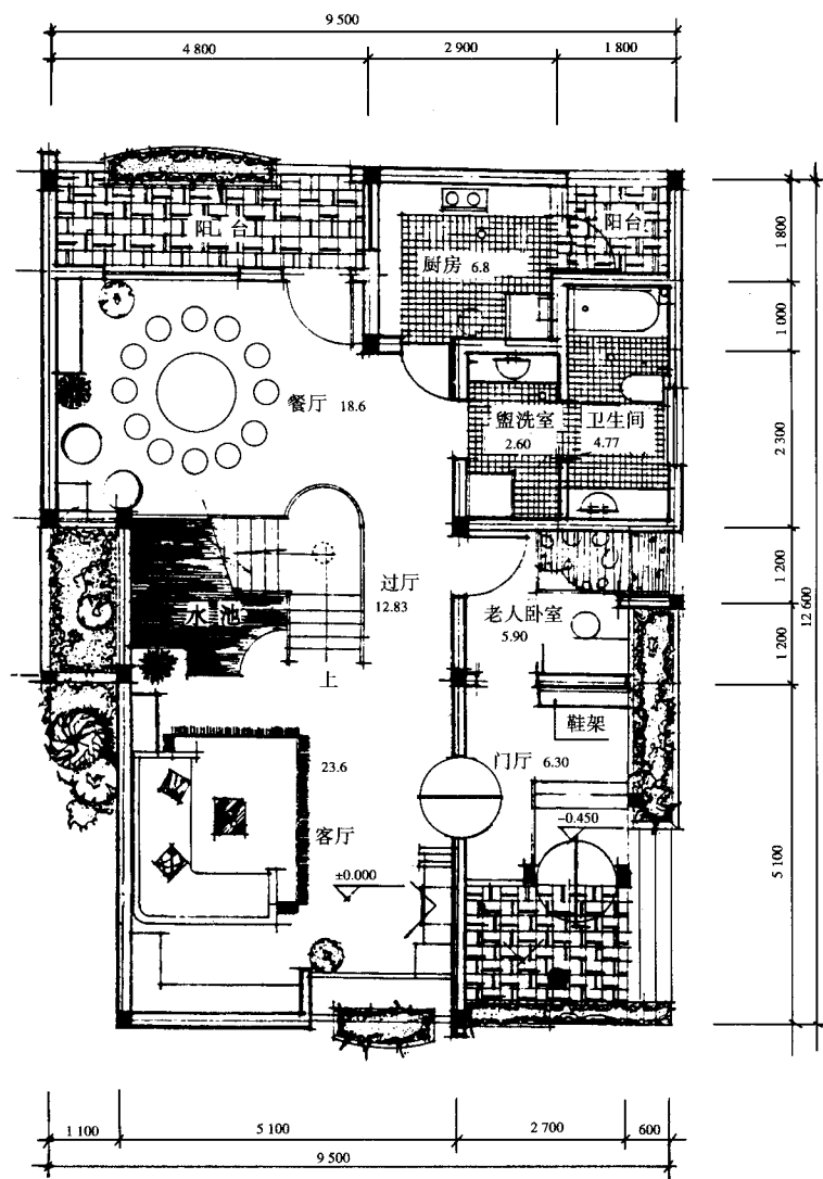
底层平面图
