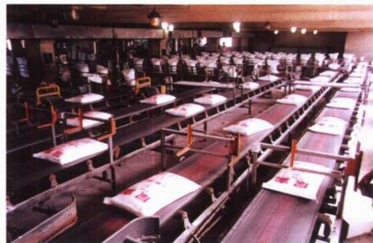
尿素包装线
