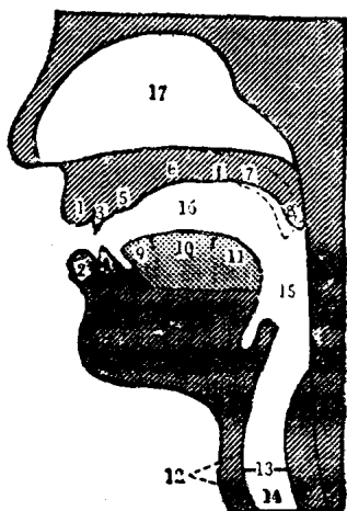
发音器官图
