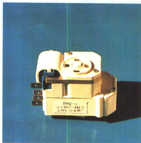
DSQ—1 冰箱自动化霜定时器
