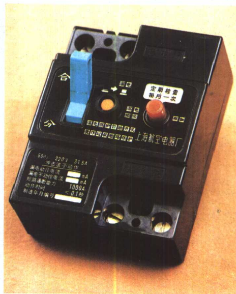
JCBI. JCB2 漏电保护自动开关系列
