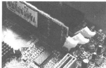
图 1-3 内存旁的塑料卡子没有固定好
