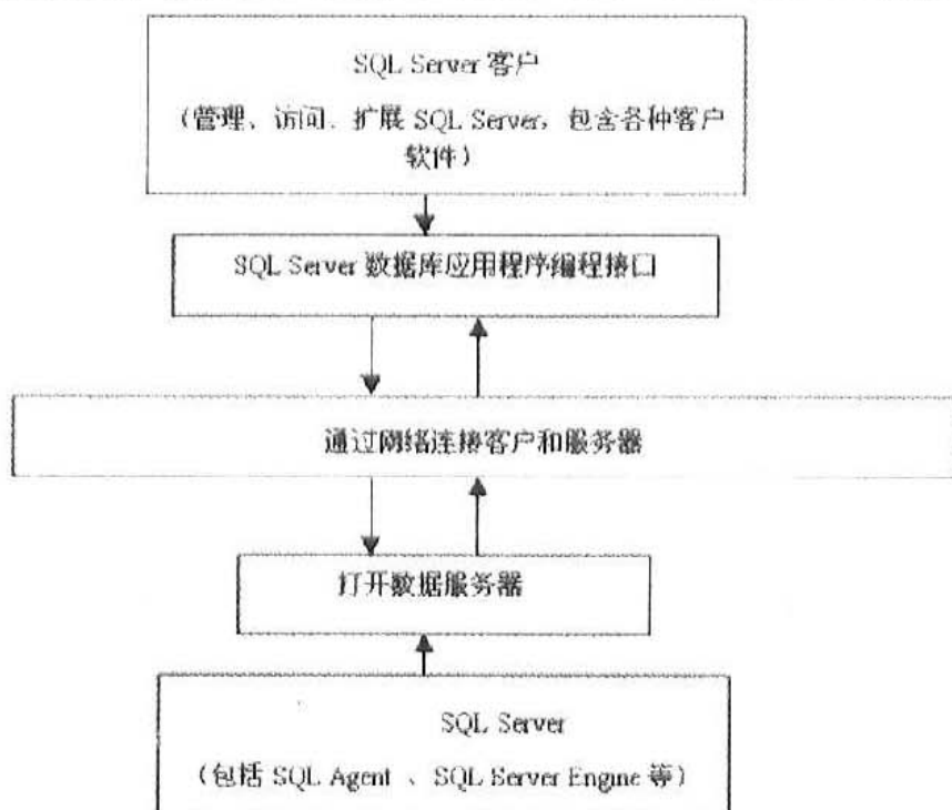
图 1-2 SQL Server 客户/服务器结构
