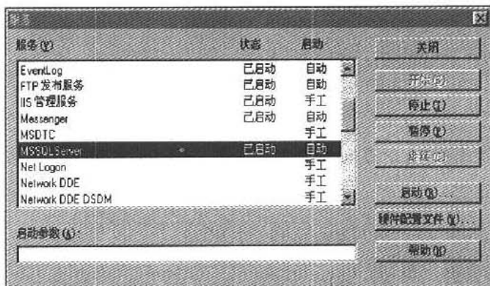
图 2-8 “服务”对话框
