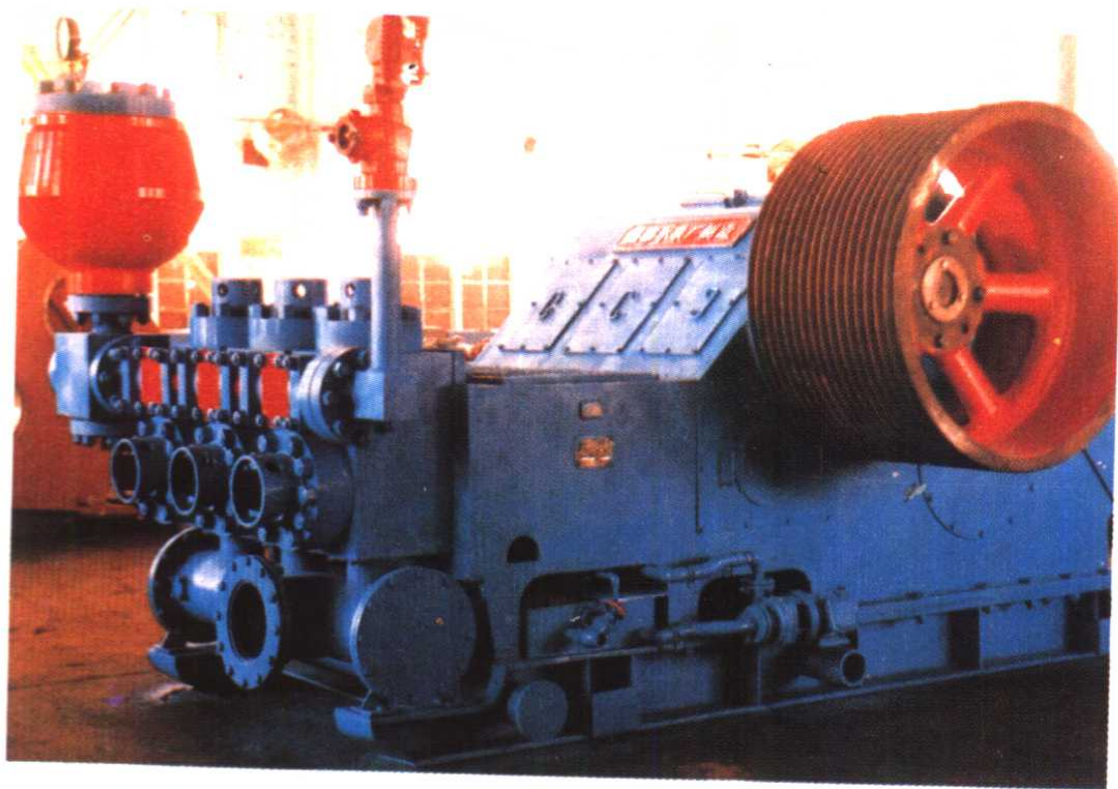
SL 3 NB - 1600A型石油泥浆泵
