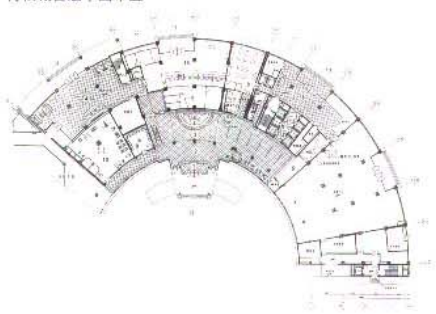
青松城首层平面布置
