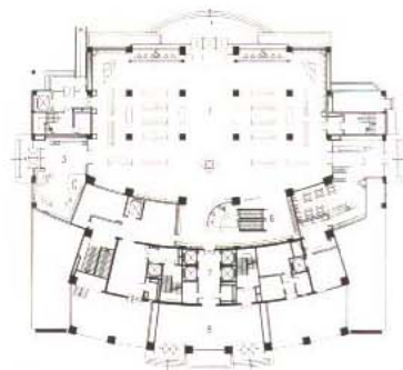
四层平面
