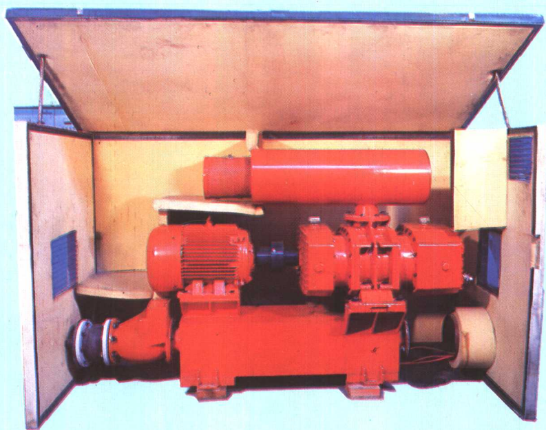
低噪声密集成套型罗茨鼓风机
