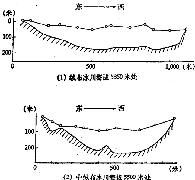
图 2 绒布冰川重力测量横剖面图
