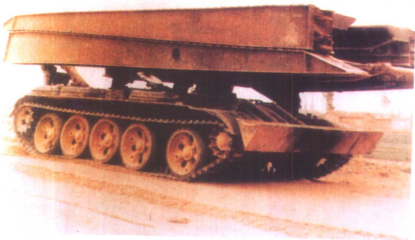
中国坦克架桥车
