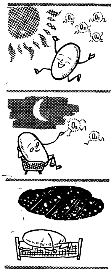
图4 微生物对各种环境的适应
