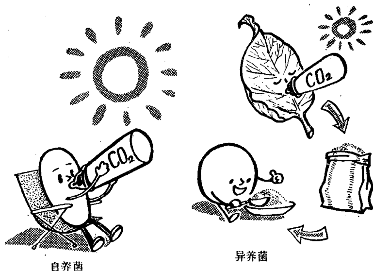
图6 自养菌与异养菌
