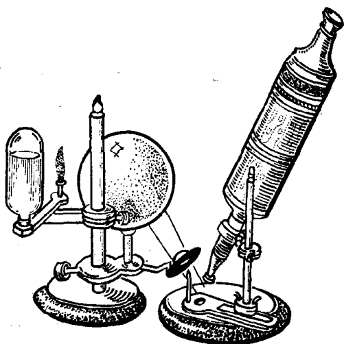
图1 最早使用的显微镜
