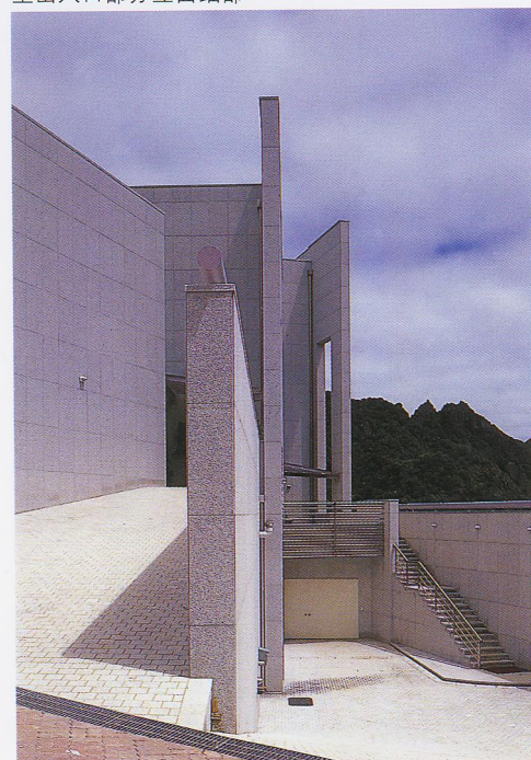
主出入口部分立面细部
