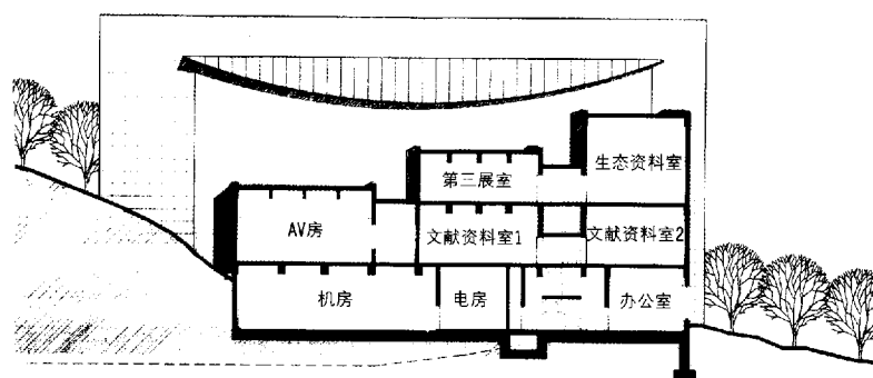
横剖面图
