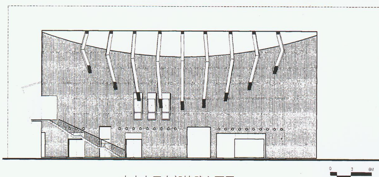
中央大厅内部墙壁立面图
