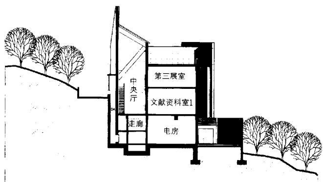
纵剖面图
