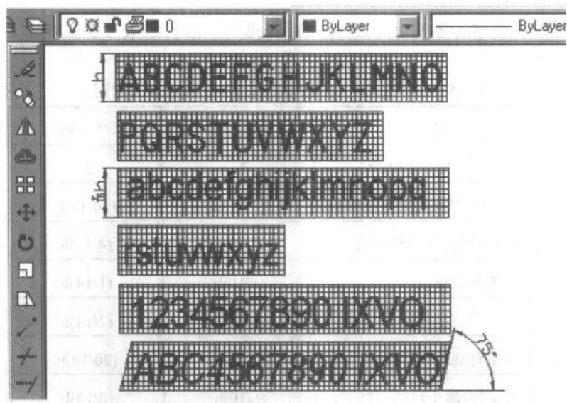
图 1-8 字母和数字的窄字体
