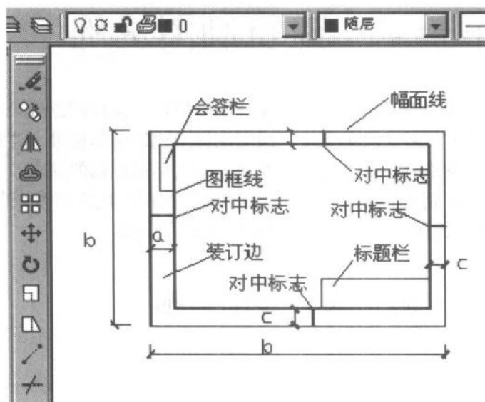
A0~A3 横式幅面
