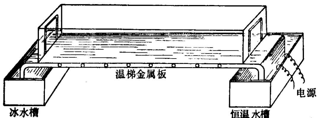
图 2-1 温度等级器
