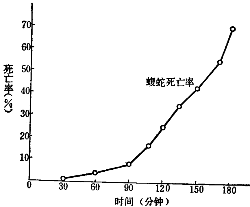
图 1-2 在 40°C 条件下,蝮蛇死亡率与忍受时间的关系
