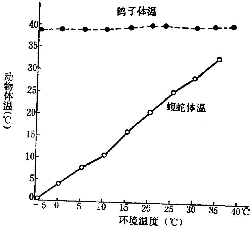
图 1-1 动物体温与环境温度的关系
