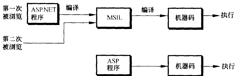
图 1-3 ASP 和 ASP.NET 编译方式的比较
