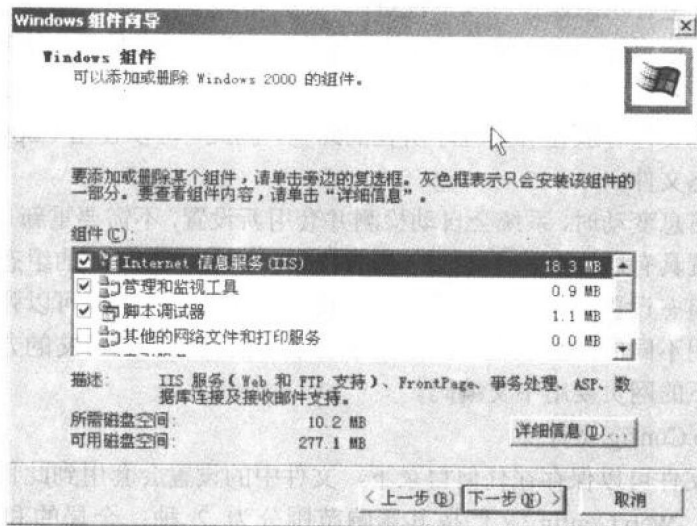
图 1-5 安装 IIS 5.0
