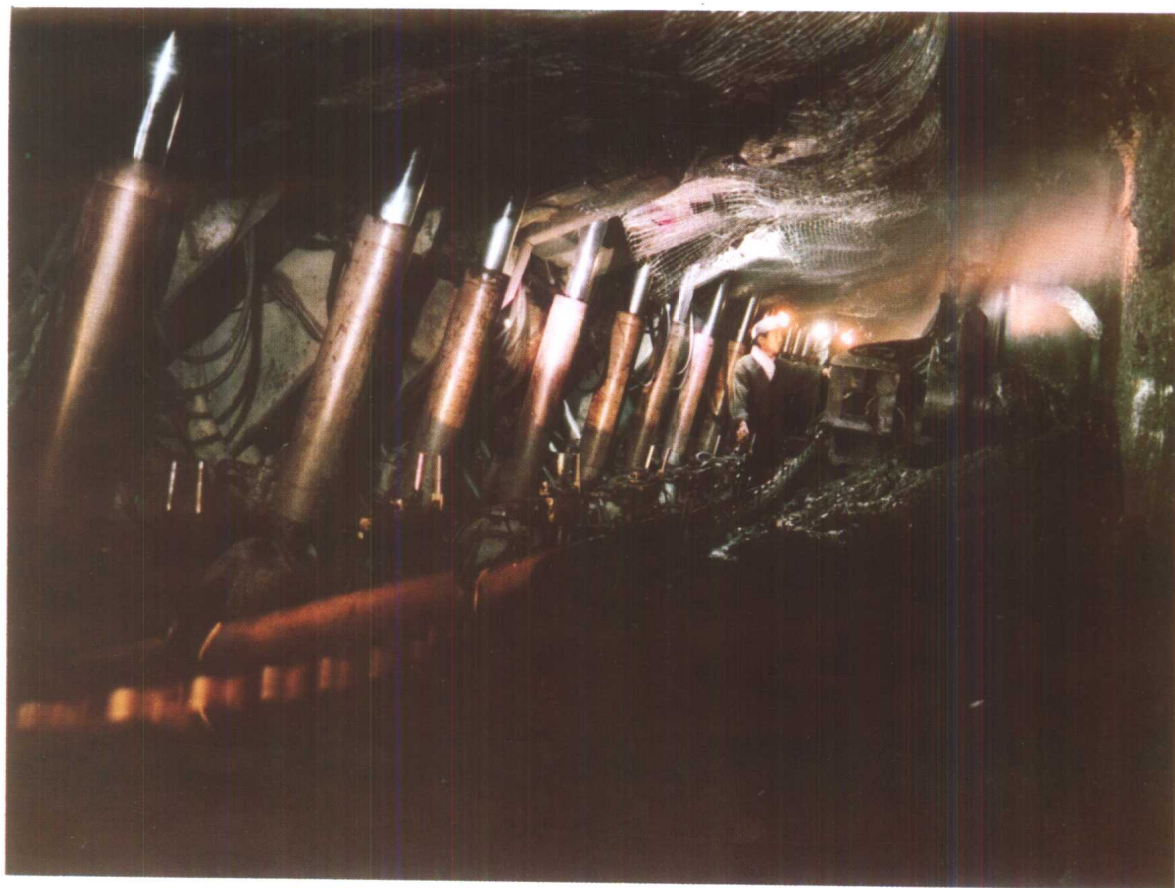
河南平顶山矿务局一矿井下综合机械化采煤工作面
