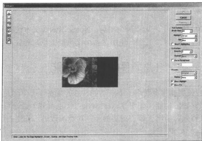
图 1-15 Extract 对话框
