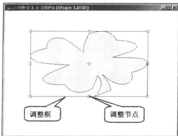
图 1-14 调整框
