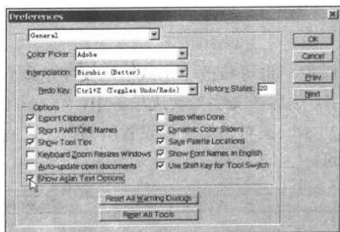
图 1-9 Preferences 对话框
