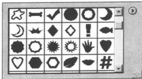
图 1-3 “形状”列表框
