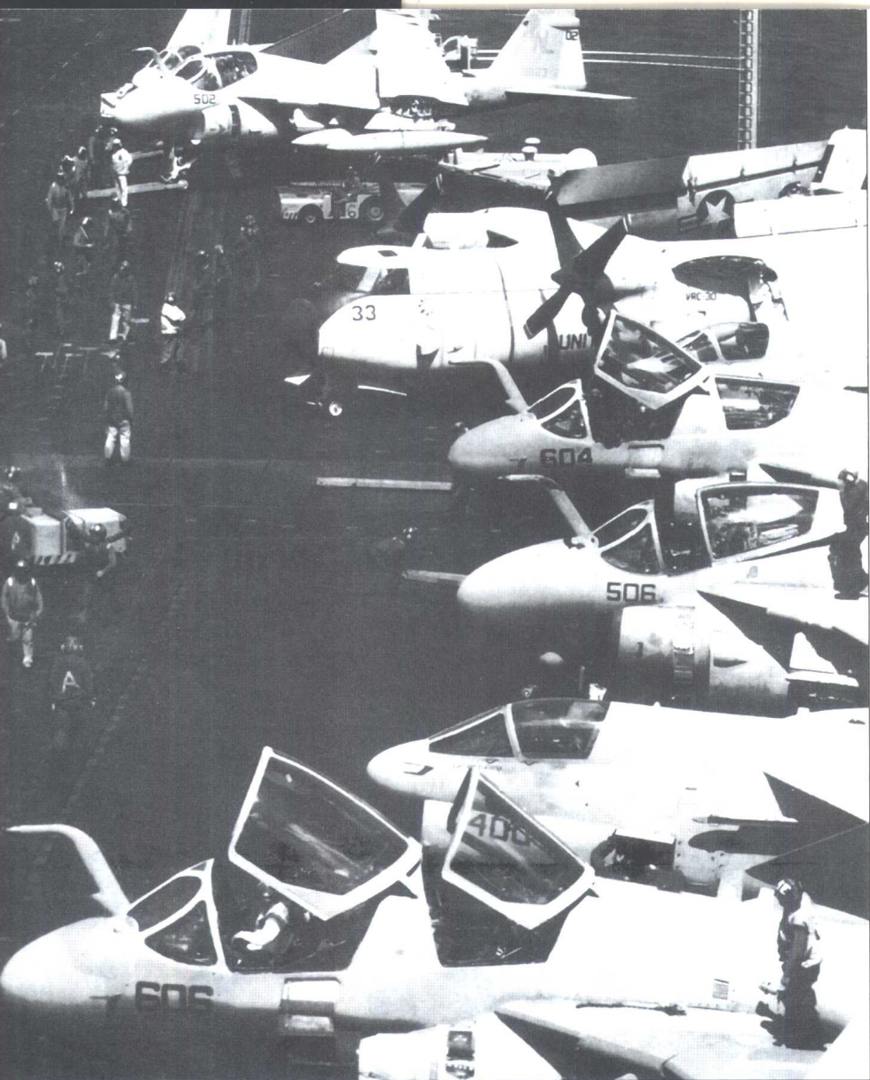
繁忙的航母甲板。照片最下部606机即是“徘徊者”飞机，可以清楚地看到它的前后2个座舱和机头伸出的空中加油探管。
