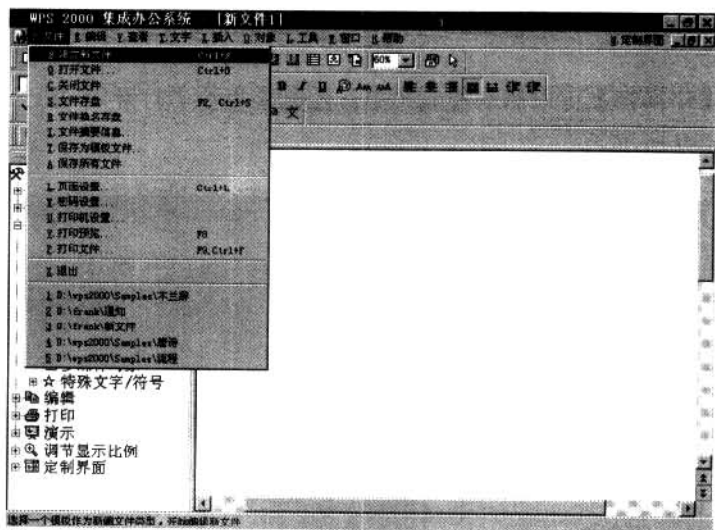
图 2-10 “文件”菜单
