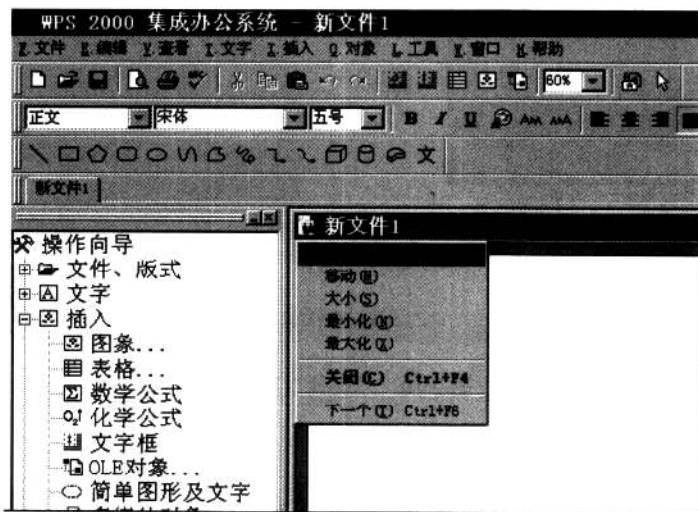
图 2-9 控制菜单
