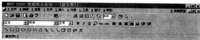
图 2-11 工具栏
