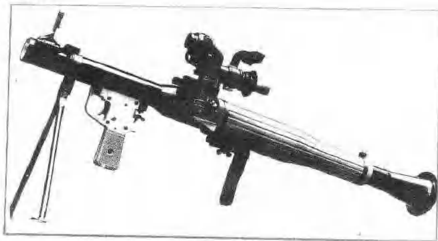
9307厂生产的69式40毫米火箭筒
