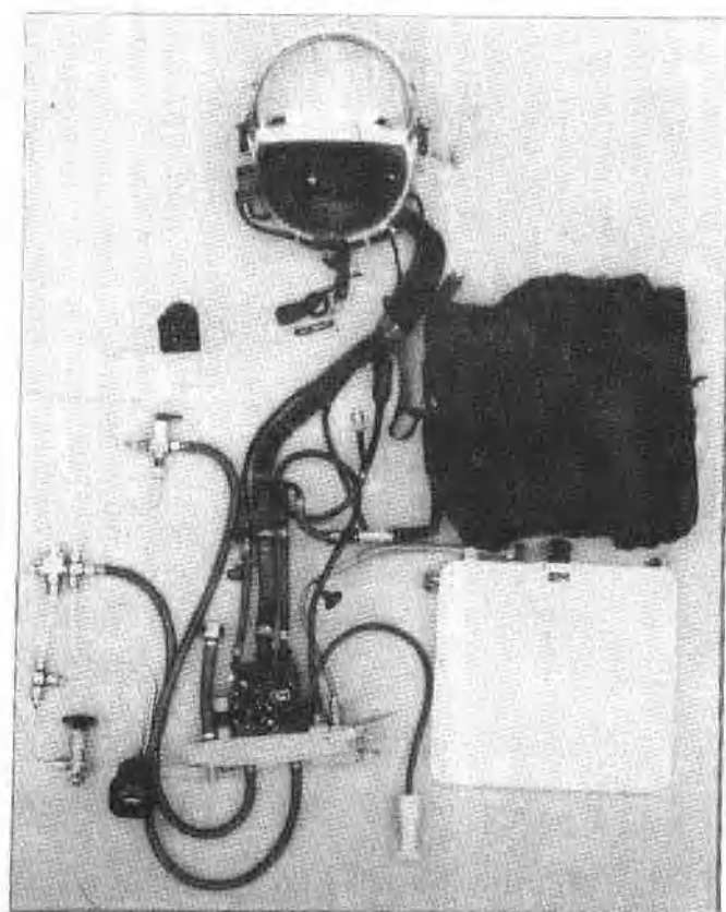
351 厂研制的航空供氧系统
