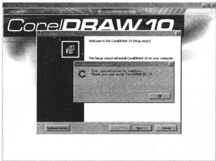
图 1-13 安装完成
