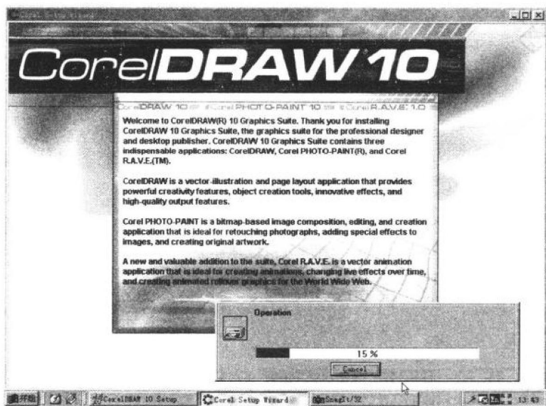
图 1-12 文件复制
