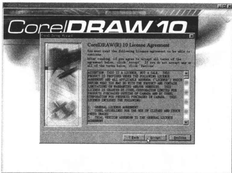
图 1-3 服务协议
