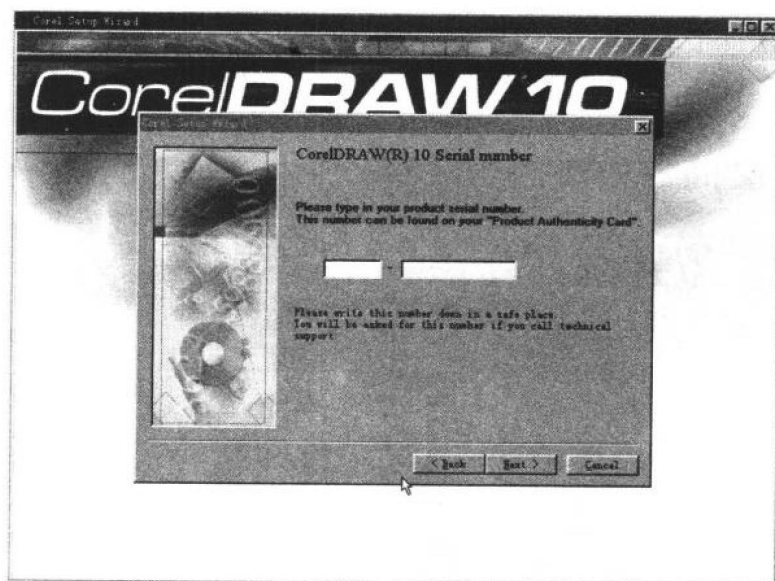
图 1-5 输入序列号
