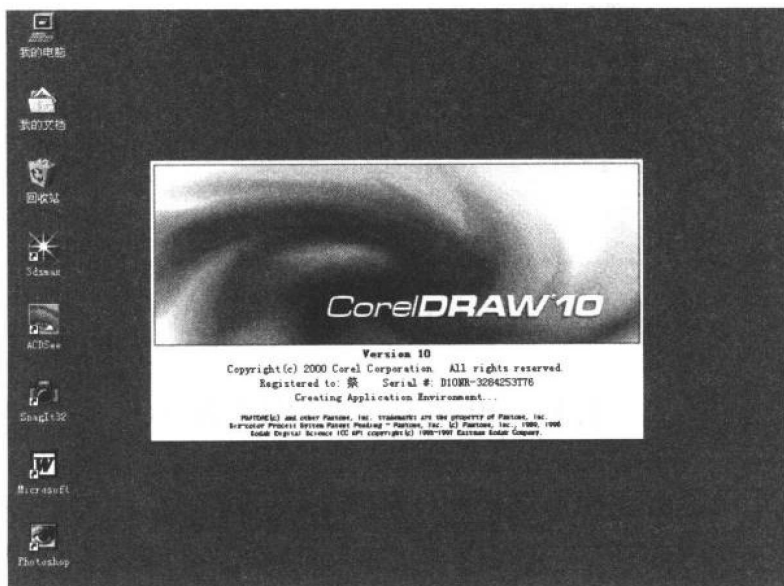
图 1-14 启动画面
