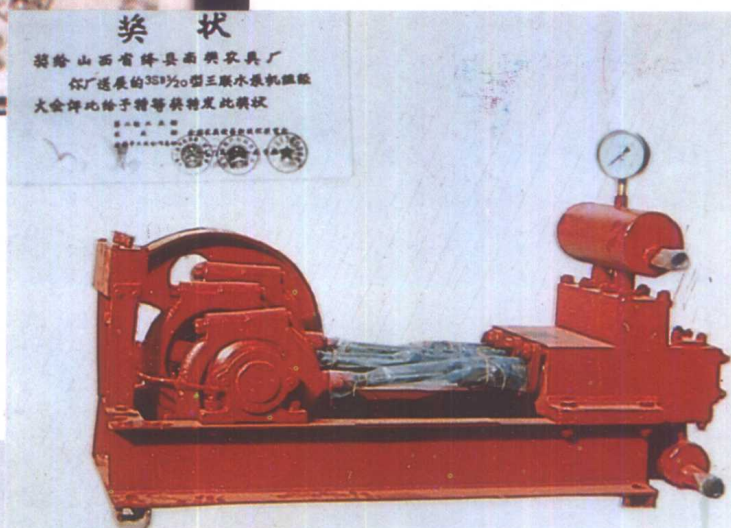
县南樊机械厂生产的三 联泵在全国获得的奖状
