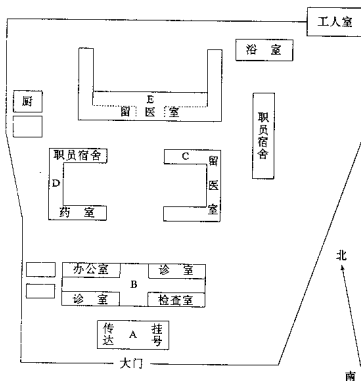
桂林市政府工务科测绘地盘图
