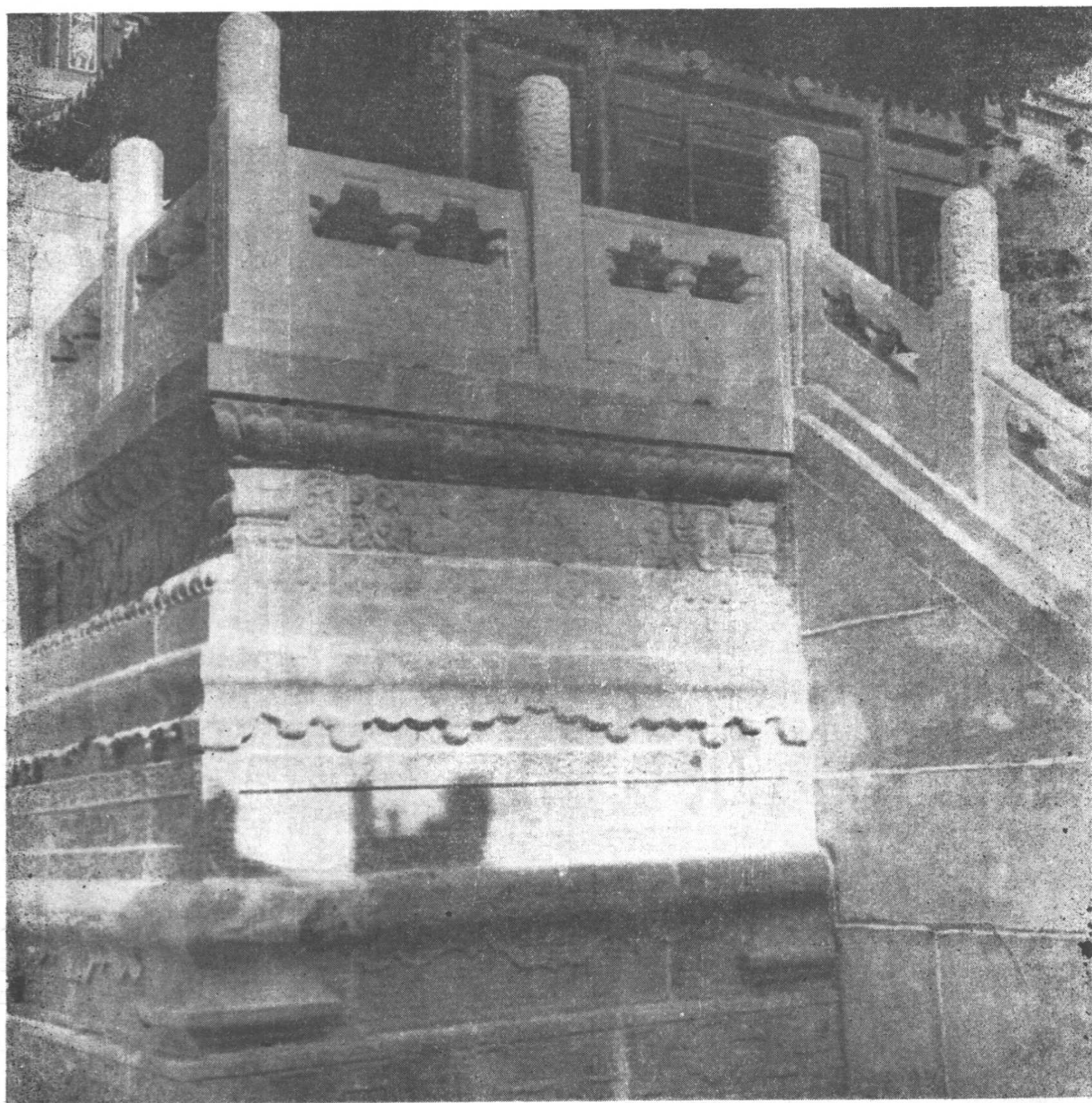
北京頤和園銅亭兩層須彌座台基及石欄杆
