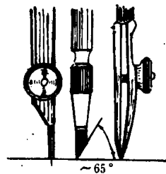
图 1-12 圆规两腿应高低一致
