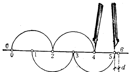
图 1-11 用分规等分线段
