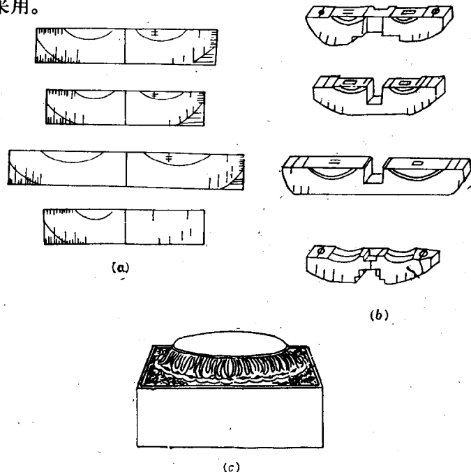
图1 《营造法式》中图样举例 (a) 斗拱斗口正投影图；(b) 斜轴测图；(c) 柱脚透视图
