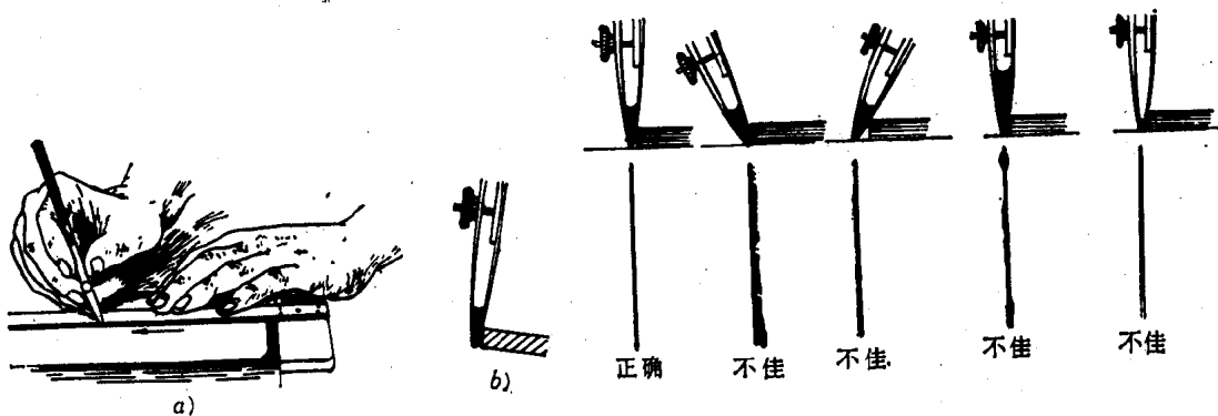
图 1-20 墨线易出现的弊病
