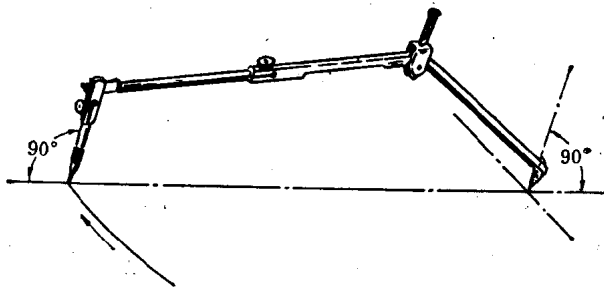
图 1-16 圆规加添加长杆画大圆
