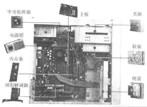
图 1.3.3 主板示意图
