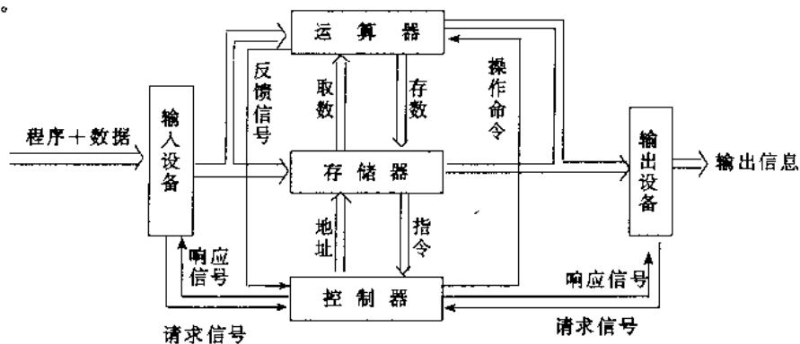
图 1.2.2 计算机硬件结构框图
