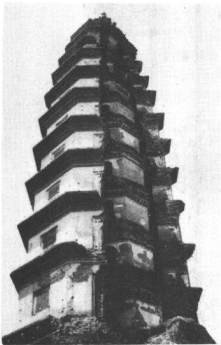
图十一 定县开元寺料敌塔东侧立面
