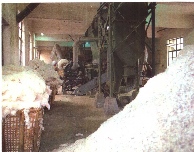
余姚市供销合作社泗门棉花加工厂
