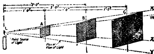
第四圖 光之傳播
