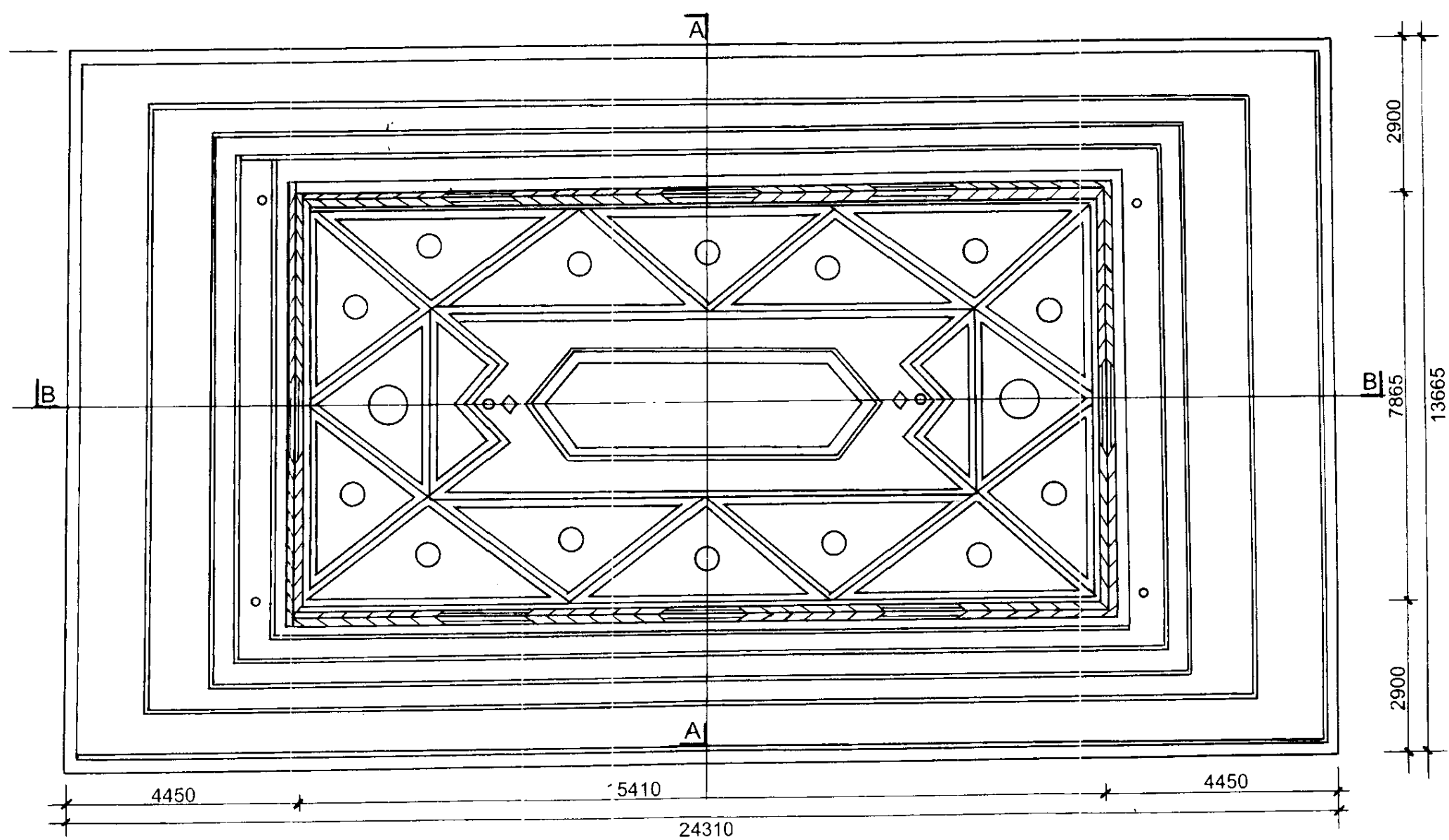
顶棚平面图
