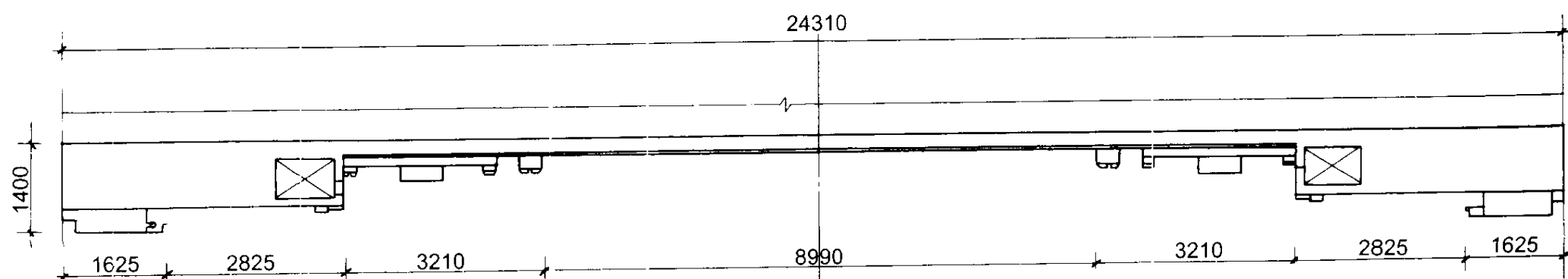
B-B剖面图
