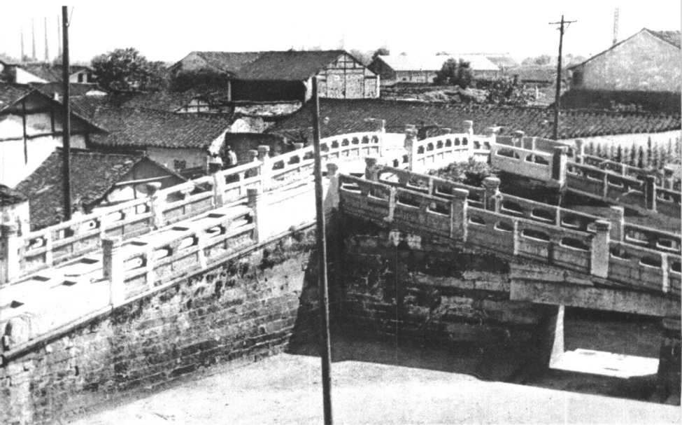
②③ 绍兴八字桥
