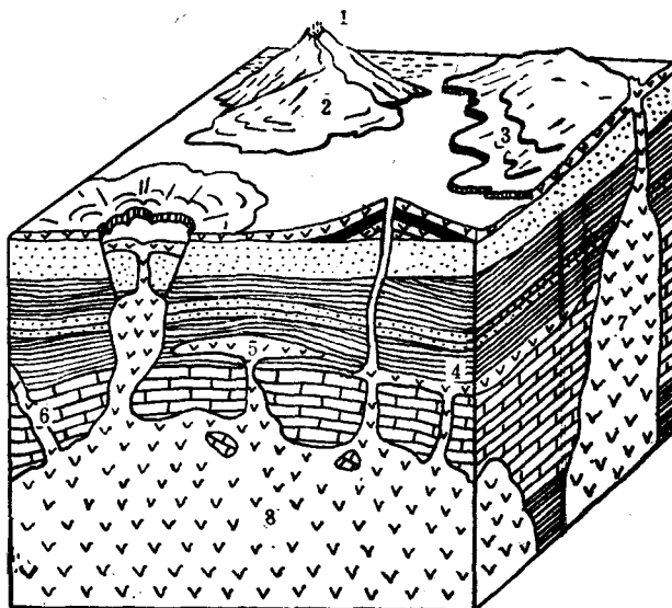
图1-3 岩浆侵入体和喷出体示意图
