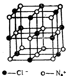
图1-1 食盐晶格构造
