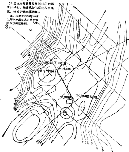
附图1: 大同县长垣湖 的地震构造图
