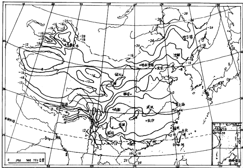
一月平均气温分布图 (°C)
