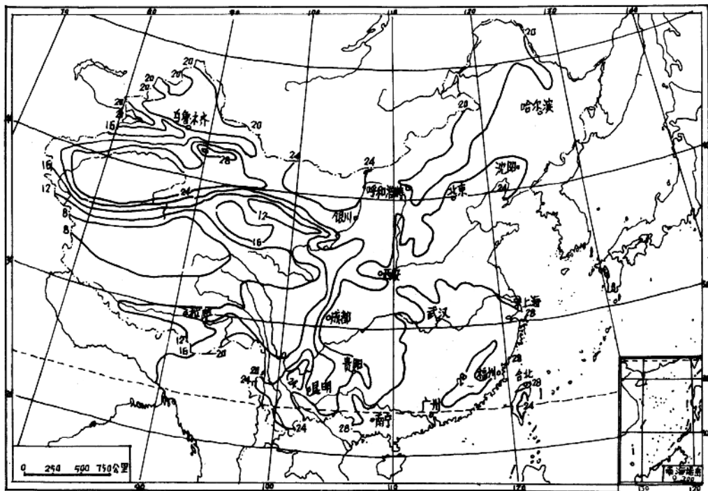
七月平均气温分布图 (°C)
