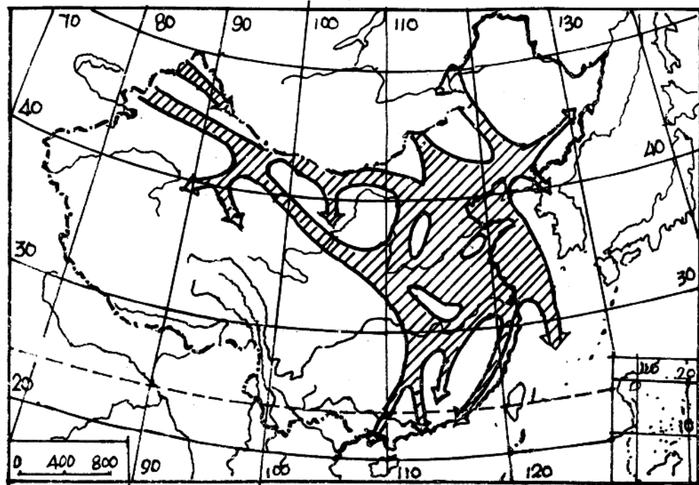
中国境内寒潮路径示意图
