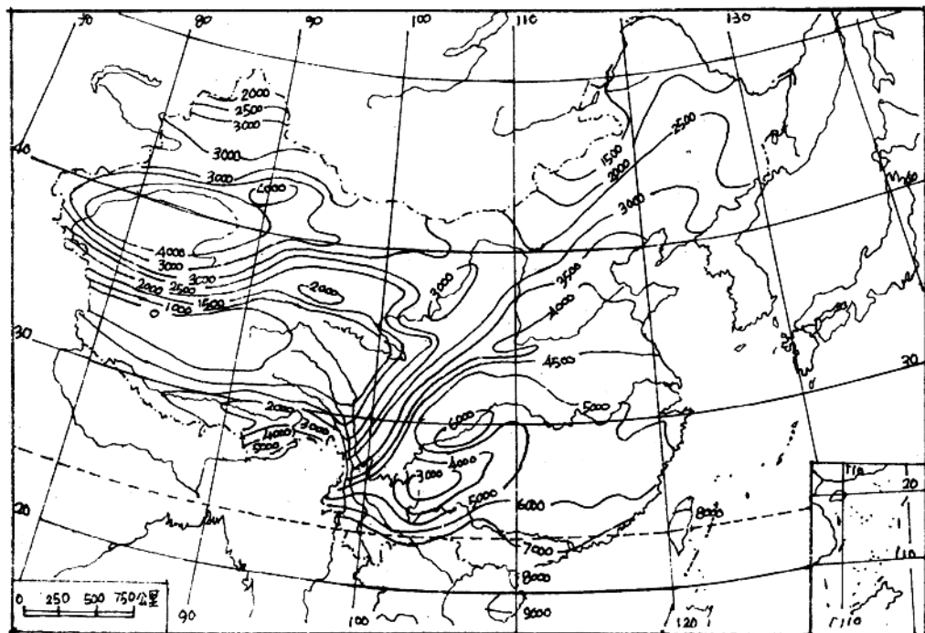
中国日平均气温 \geq 10^{\circ}\text{C} 稳定期积温 ( ^{\circ}\text{C} )
