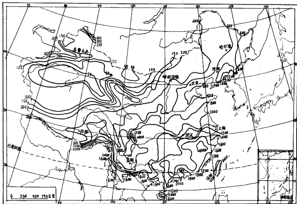
中国年降水量分布图
