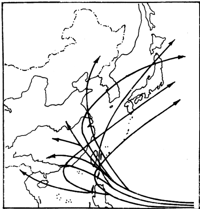
中国台风移动路径示意图
