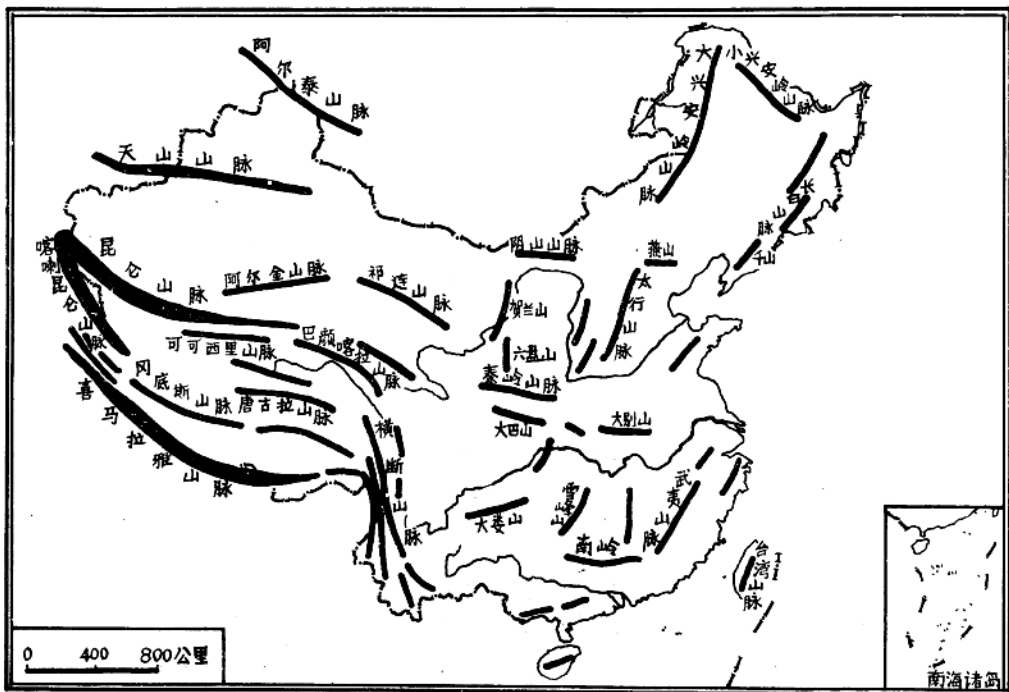
中国主要山脉图
