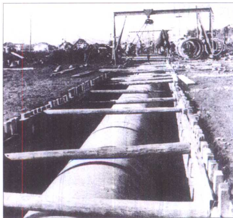
施工中的污水干管(1985 年)
