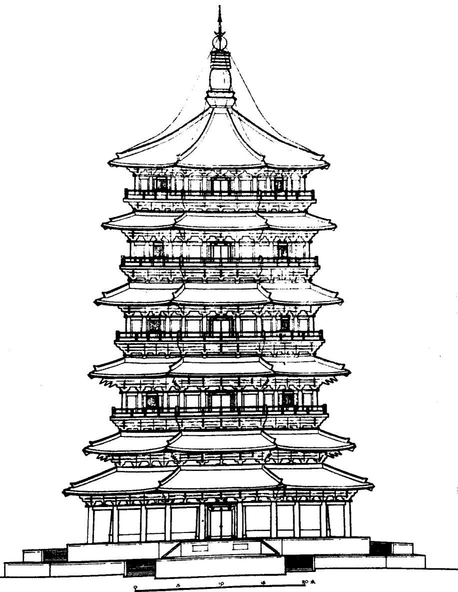
木塔南面立面图 陈明达绘
