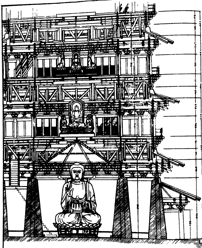
第一至四层平坐断面图 陈明达绘
