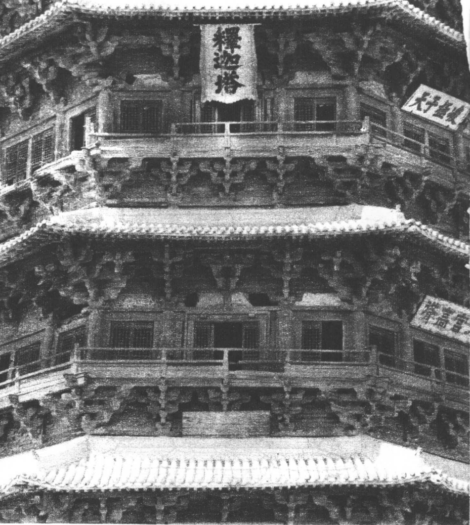
第一至三层东南面外景
