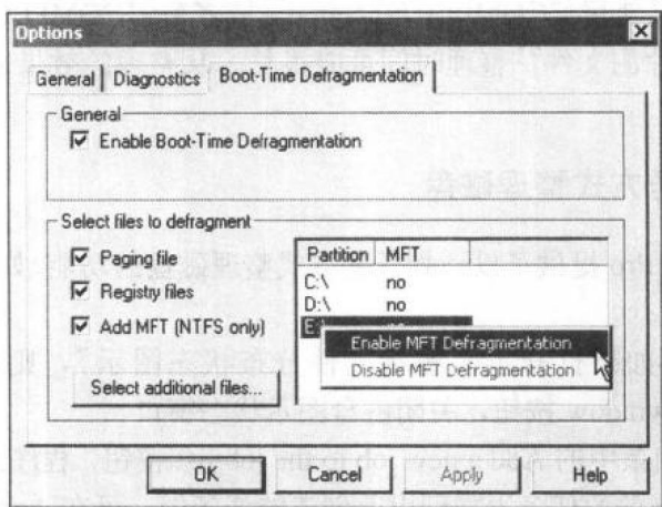
图 1-6 Boot-Time Defragmentation 设置界面
