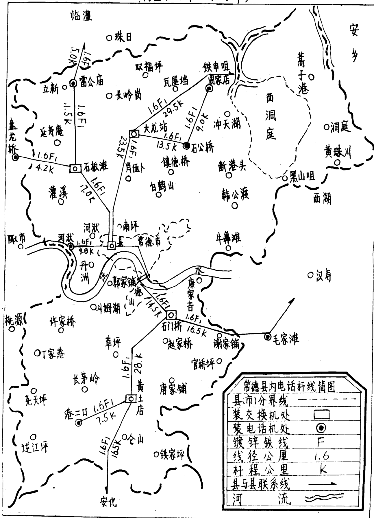
常德县内电话线路(示意图一) 民国十八年(1929年)
