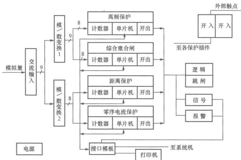
图 1-3 多 CPU 结构的微机继电保护装置硬件框图
