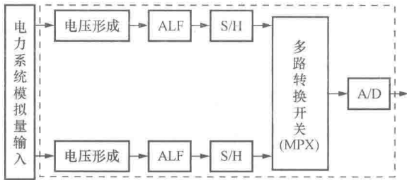
图 1-6 逐次逼近原理 A/D 数据采集系统构成框图
