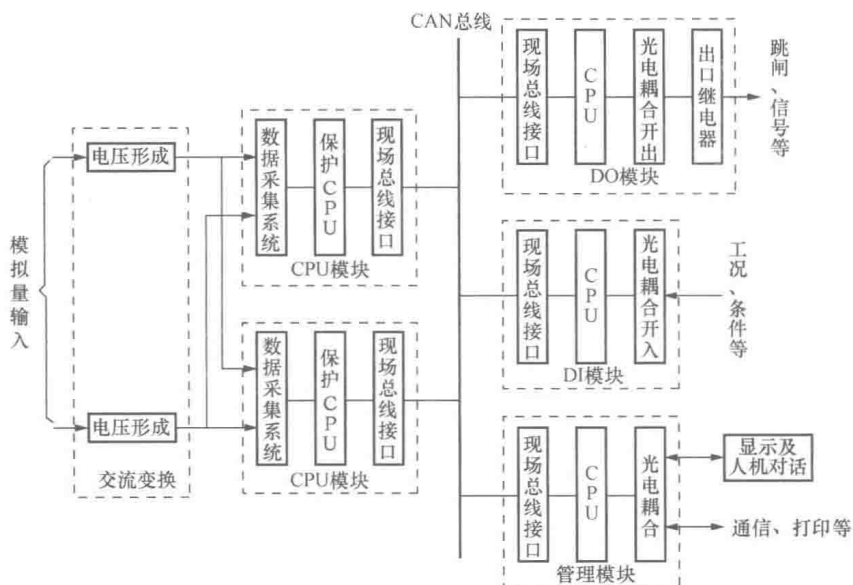
图 1-5 网络化的微机继电保护装置典型硬件框图
