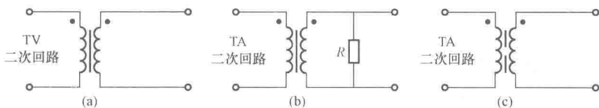
图 1-7 输入变换及电压形成回路的原理图
