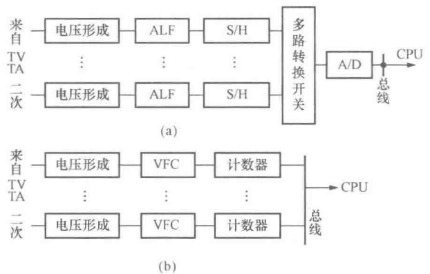
图 1-2 模拟量输入回路框图
