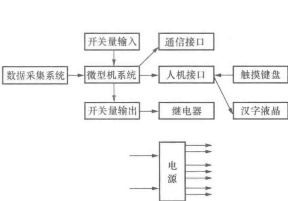
图 1-1 典型微机继电保护装置硬件系统结构
