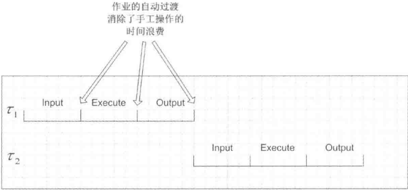
图 1-3 单道批处理系统的任务运行
