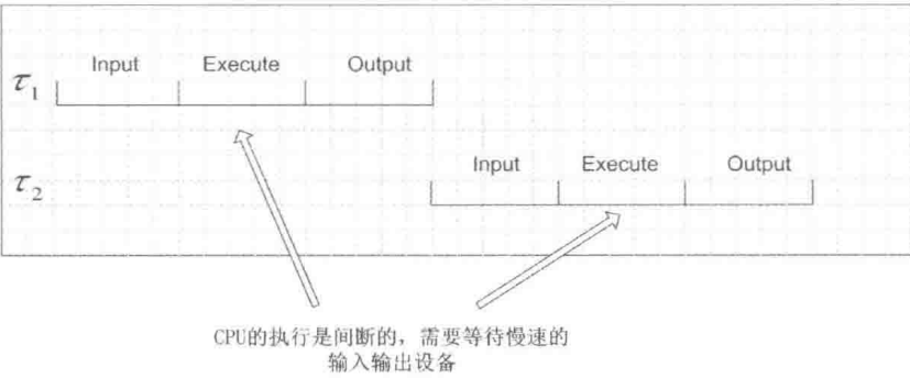
图 1-4 单道批处理系统的问题
