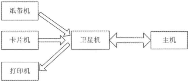
图 1-5 卫星机的运行
